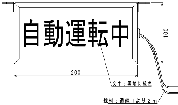
下部取付時
