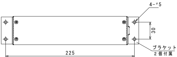
下部取付時
